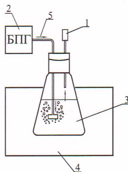
Рис. 3. Устройство для концентрирования на сорбент: 1 – адсорбционная ловушка с сорбентом; 2 – блок подготовки газов; 3 – анализируемая вода; 4 – водяная баня; 5 – направление потока.
